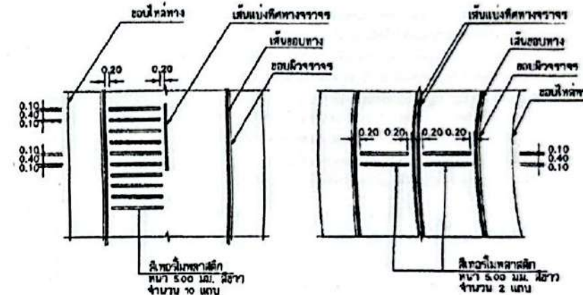
แบบขยาย A RUMBLE STRIPS
