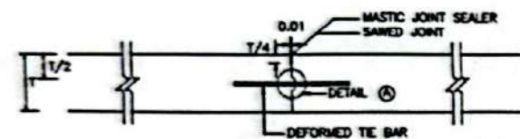
LONGITUDINAL JOINT
