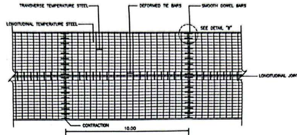
แบบแสดงการเสริมเหล็กแบบ ค.ส.ล.
