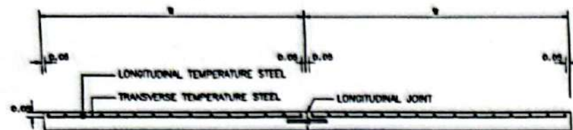
รูปตัดตามขวาง ๑๖๖๖๖๖ ค.ส.ล.
