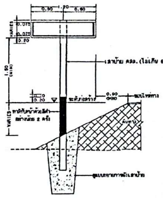
แสดงการปักเสาป้ายหน้า N-1 และ N-4
