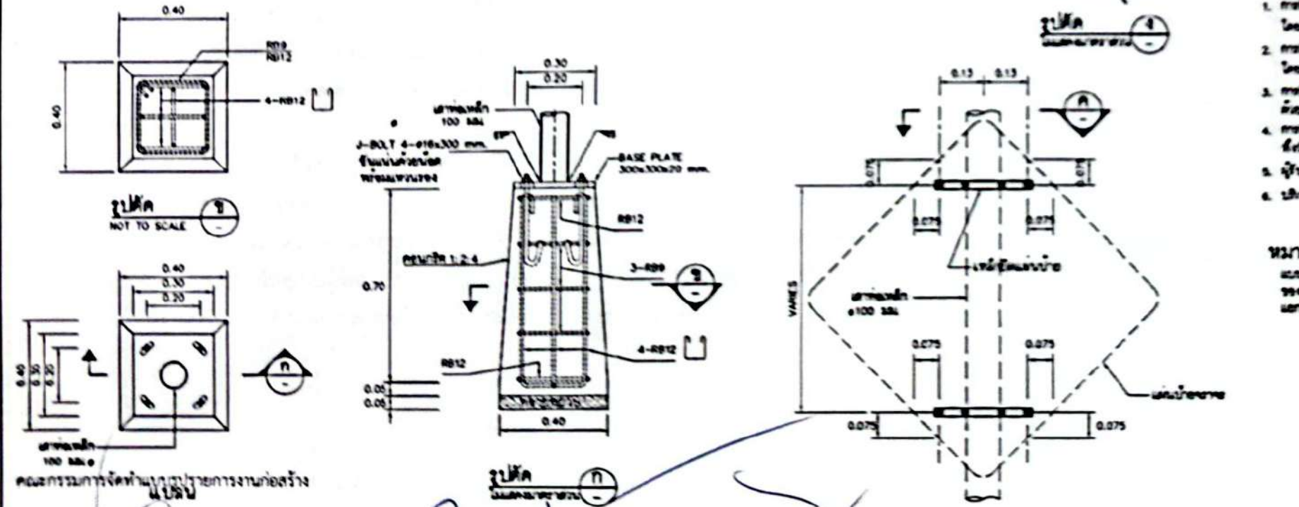
ไฟกะพริบ รูปด้านหน้า ไฟกะพริบร่วมกับป้ายจราจร แสดงการติดตั้งสัญญาณไฟกะพริบอย่างเดียวหรือร่วมกับป้ายบังคับหรือป้ายเตือน (เสาหลัก) แบบมาตรฐาน
