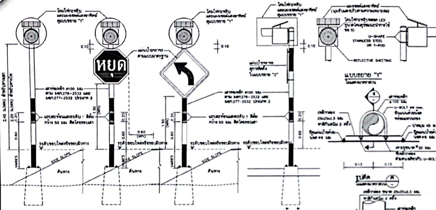
ไฟกะพริบ รูปด้านหน้า ไฟกะพริบร่วมกับป้ายจราจร แสดงการติดตั้งสัญญาณไฟกะพริบอย่างเดียวหรือร่วมกับป้ายบังคับหรือป้ายเตือน (เสาหลัก) แบบมาตรฐาน
